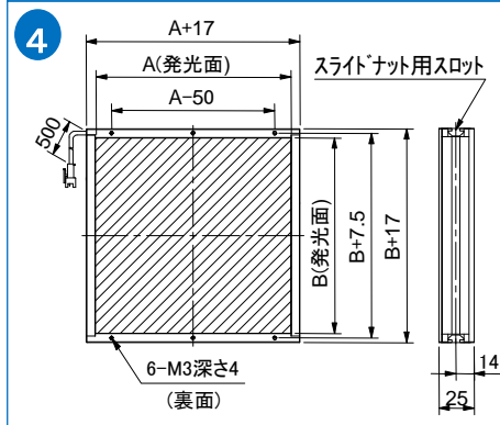
スライドナット用スロット
