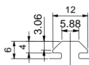
スライドナット用スロット
